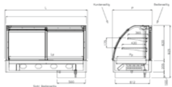
Vermaßungsskizze Zentralkühlung
